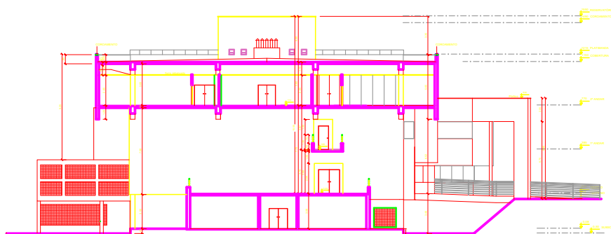
CORTE T1
