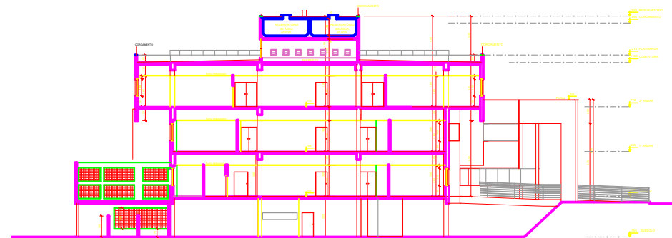
CORTE T2
