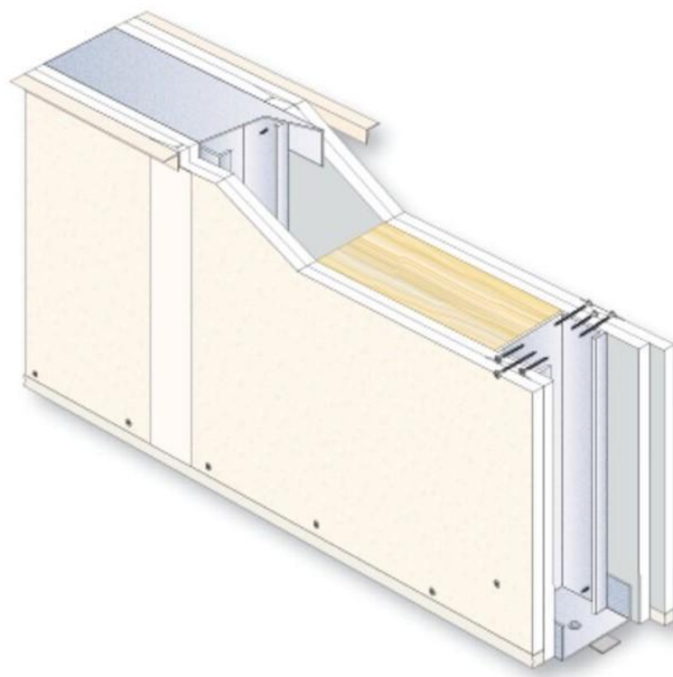
Figura 1- Parede divisória
